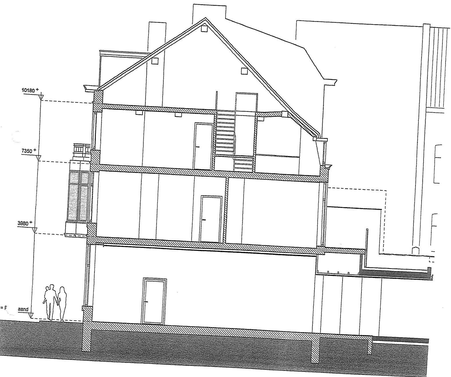
DOORSNEDE A-A
