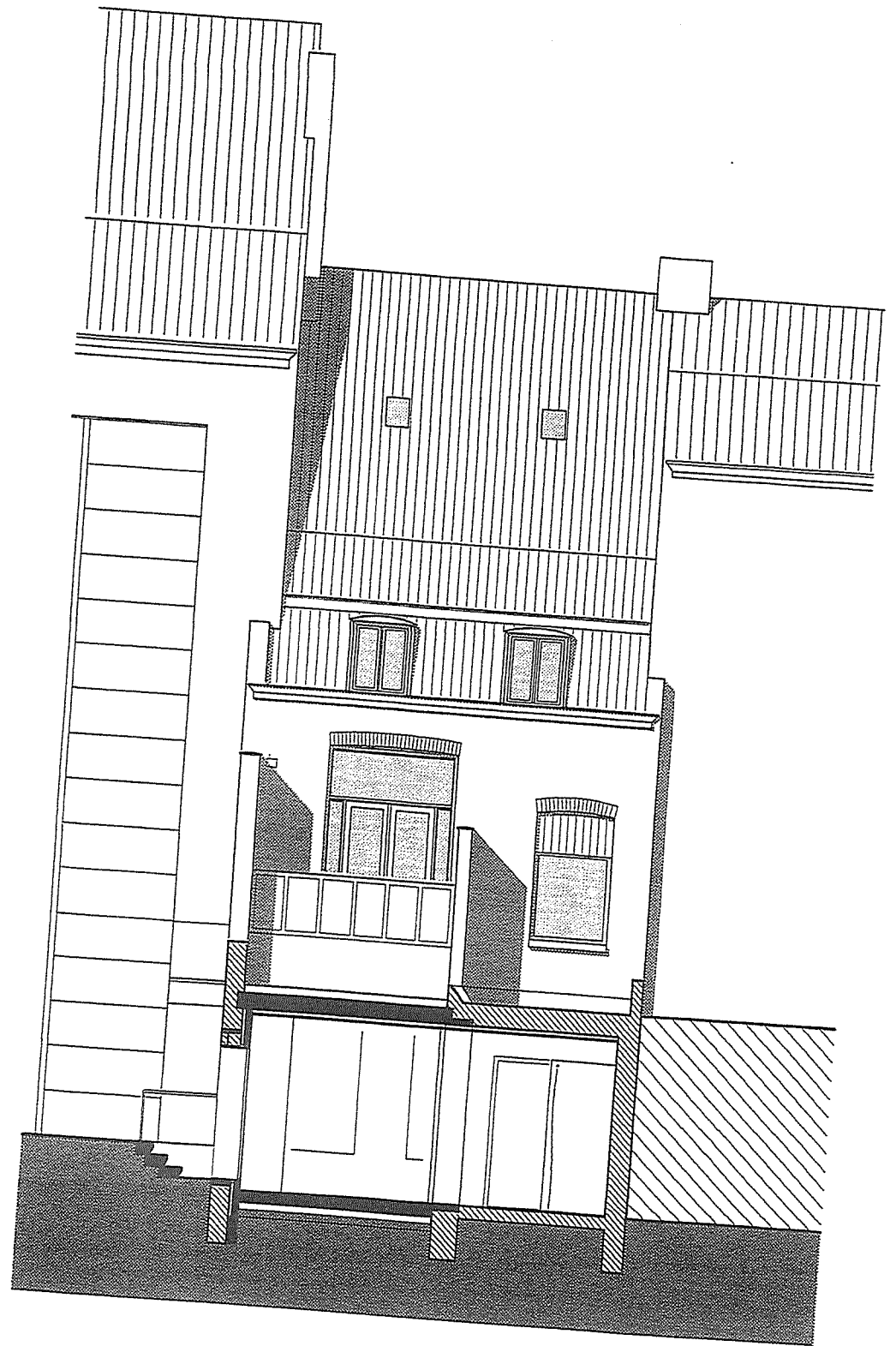
ACHTERGEVEL
